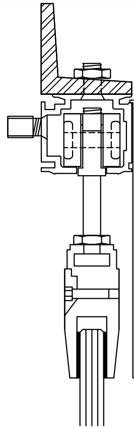
1 DOOR HEADER SECTION SCALE : 6"=1'-0"
